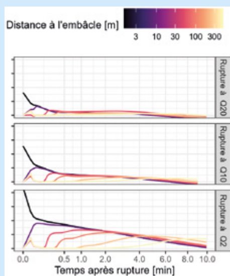
Hauteur de l'onde de rupture de l'embâcle du Taurou estimée par simulation numérique pour différentes hypothèses de débit de rupture (Q2, Q10 & Q20) : a) profil en long de la hauteur le long du chenal estimé à différentes durées après la rupture (0, 1, 3, 7, 12, 20 et 30 minutes) et b) évolution temporelle de la hauteur d'eau à différentes distances de l'embâcle (1, 10, 50, 100, 250 et 500 m)
