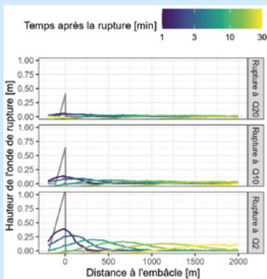
Hauteur de l'onde de rupture de l'embâcle du Taurou estimée par simulation numérique pour différentes hypothèses de débit de rupture (Q2, Q10 & Q20) : a) profil en long de la hauteur le long du chenal estimé à différentes durées après la rupture (0, 1, 3, 7, 12, 20 et 30 minutes) et b) évolution temporelle de la hauteur d'eau à différentes distances de l'embâcle (1, 10, 50, 100, 250 et 500 m)
