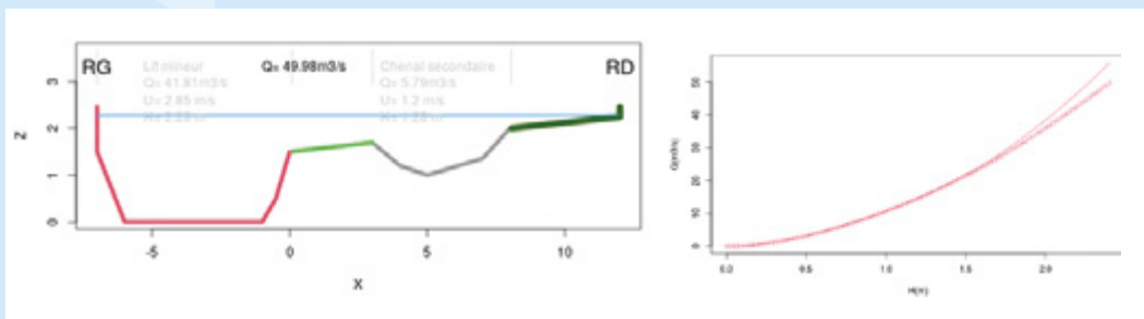
Exemples de graphes avec l'outil bedload (collaboration INRAE et OFB) : profil en travers testé et différences de hauteurs estimées avec (trait en croix) ou sans ripisylve (trait continu).
