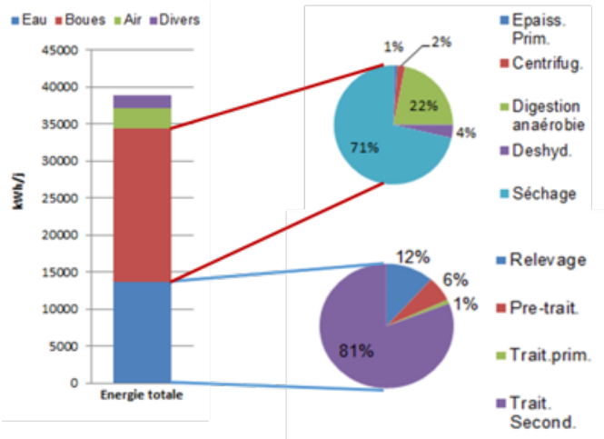
Répartition des dépenses énergétiques par file et par poste Source : Samso et al. (2017)
