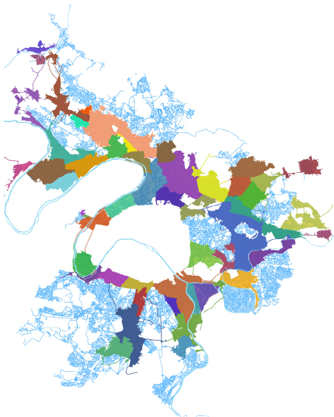
Plan de sectorisation à l'issue des études Source : SEDIF
