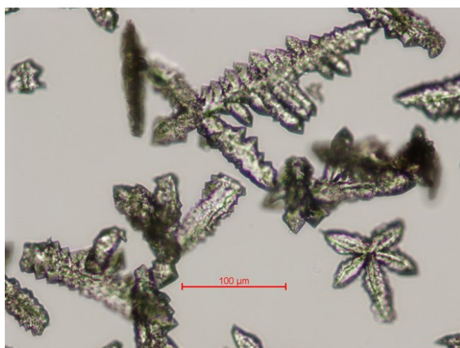
Exemples de structures à base de cristaux de struvite obtenues par précipitation du phosphore à partir du liquide issu de la bioacidification (Irstea 2018).
