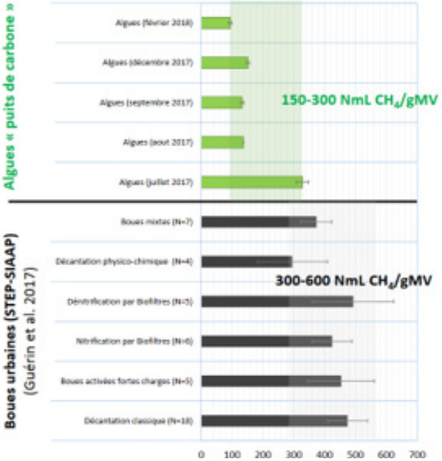
Potentiel méthanogène des algues comparé au potentiel méthanogène de boues urbaines. Source : présentation de V. Rocher, SIAAP au Congrès de l’Astee 2018
