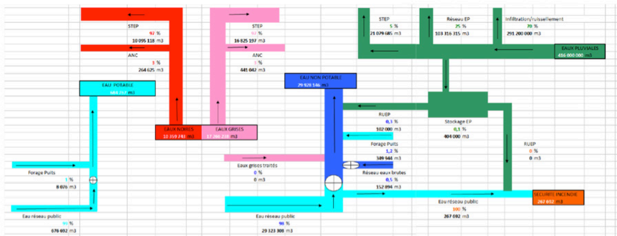
FIGURE 31 : Schéma détaillant les flux d'eau approchés de Nantes Métropole.
