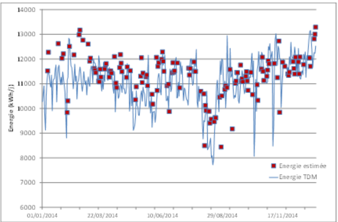
Comparaison de l'énergie modélisée et calculée à partir du temps de marche des moteurs (TDM) Source : Samso, R., Baquerizo, G., Canler, J-P., Gillot, S. (2017) Mesure et modélisation des dépenses énergétiques des stations d'épuration : vers un outil d'optimisation, 96ème Congrès de l'Astee, Liège, BEL, 6-9/06/2017
