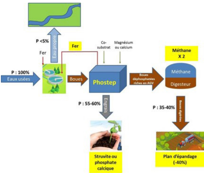
Impacts du recyclage du phosphore sur la chaîne de valorisation des boues de STEP Source : Marie-Line Daumer, Irstea
