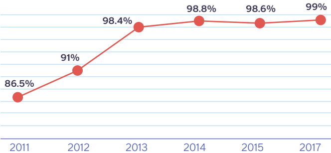
Fig. 1 : Évolution de l’autothermicité de la STEP sur la période 2011 – 2017 – Source : Biovalsan
