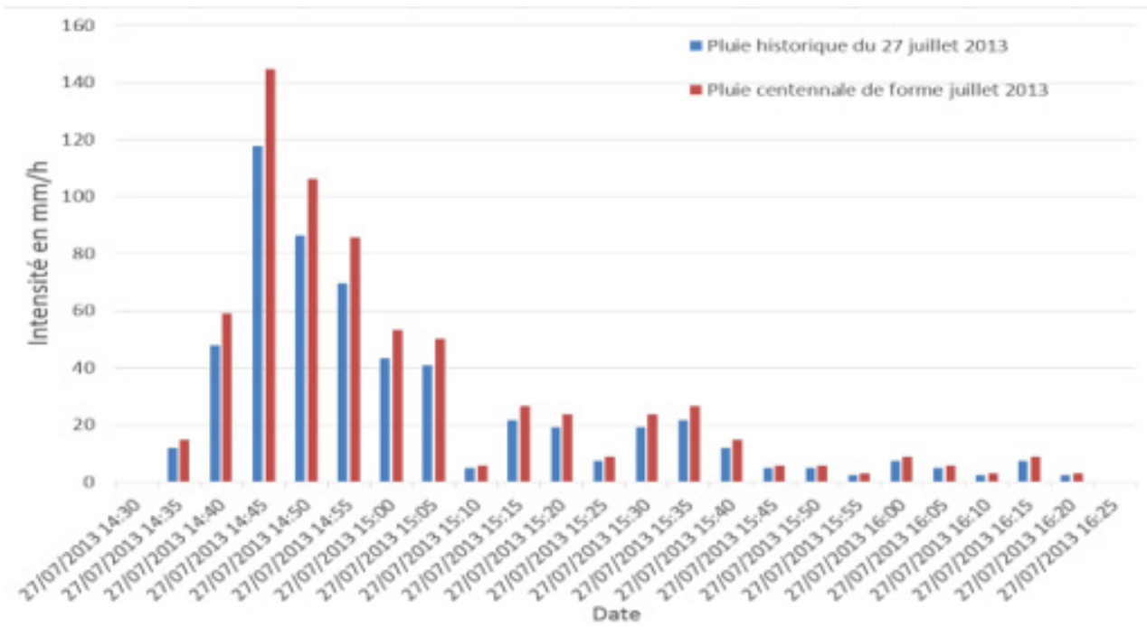
Pluie d'été centennale Source : Nantes Métropole/Prolog Ingénierie
